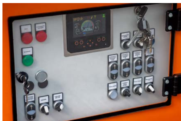
Funkcyjny pulpit sterowniczy pozwala monitorować i ustawiać parametry pracy przenośnika
